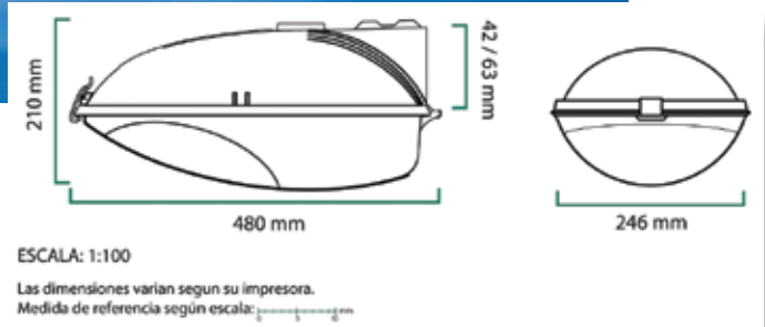
Luminaria marca Strand modelo RS 150. Medidas
