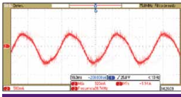
Figura 12. Corriente senoidal por la fase V del motor
