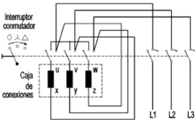
Figura 6. Esquema de conexión de un interruptor conmutador manual de estrella-triángulo
