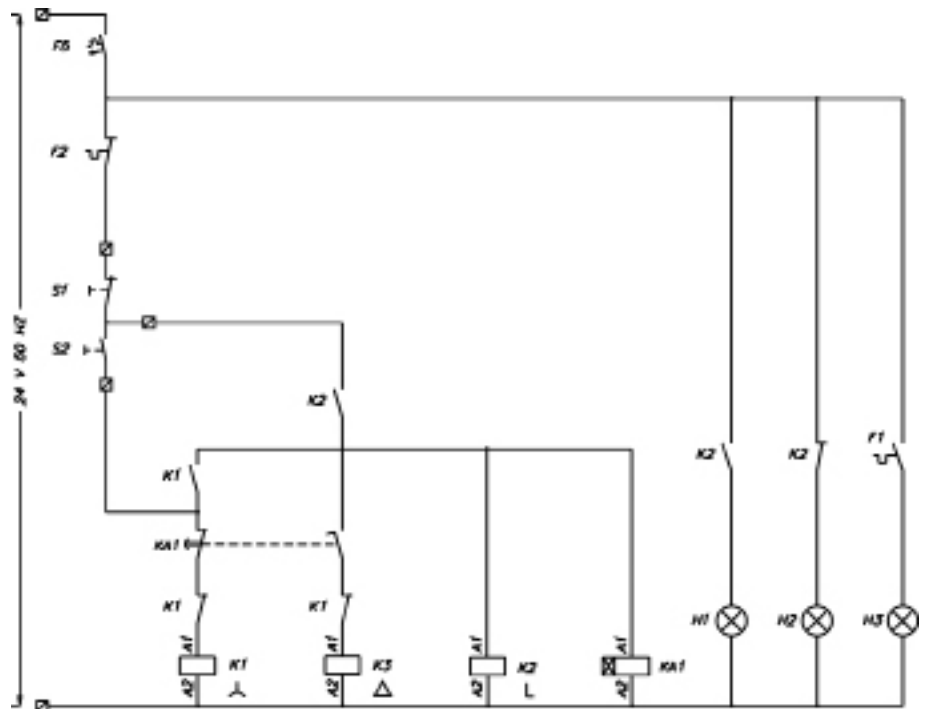
Figura 5. Circuito funcional de arranque estrella-triángulo
