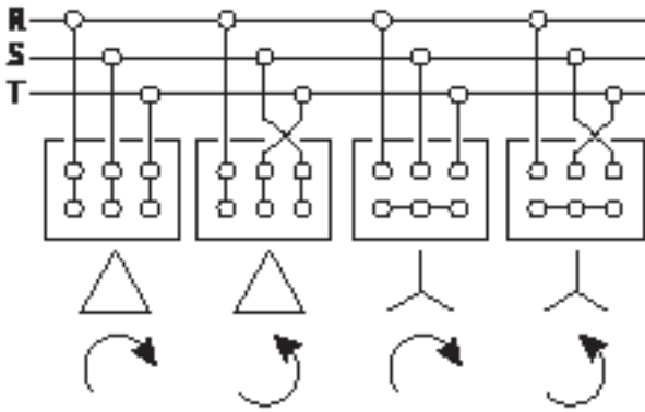
Figura 10. Sentidos de giros de motores eléctricos trifásicos
