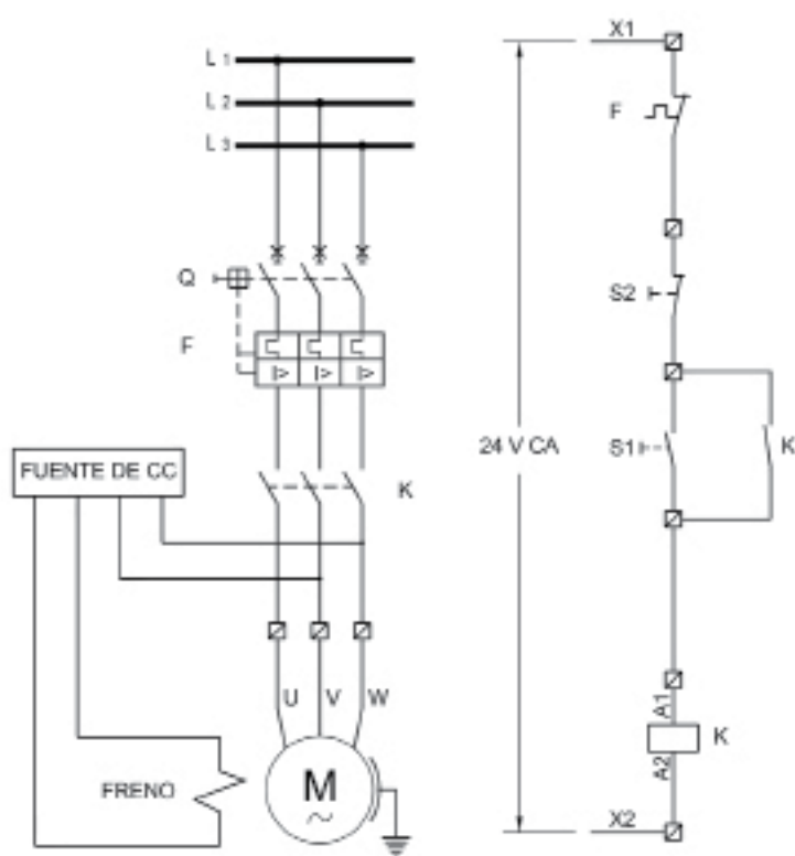
Figura 13. Esquema de frenado por corriente continua
