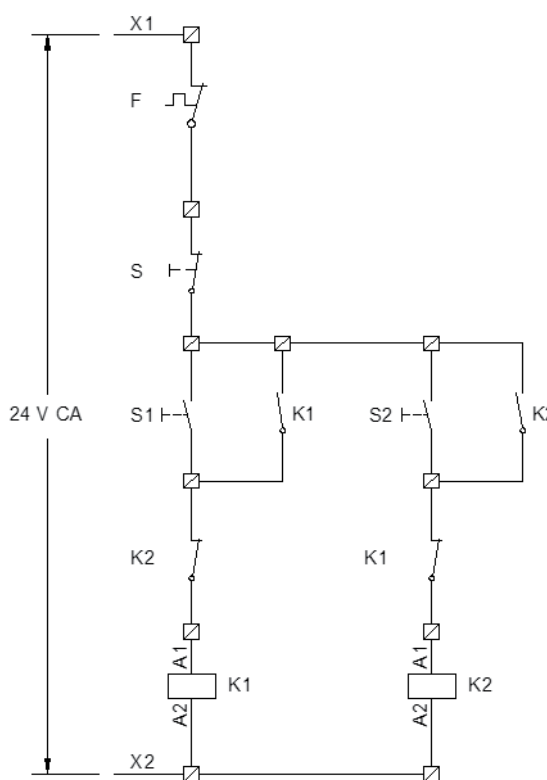
Figura 9. Circuito funcional para la inversión de marcha
