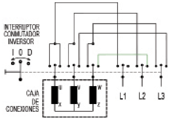
Figura 11. Interruptor conmutador manual inversor de marcha
