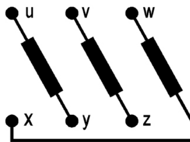
Figura 1. Bornes de las bobinas estáticas
