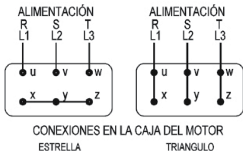
Figura 2. Esquema de conexiones de los bornes
