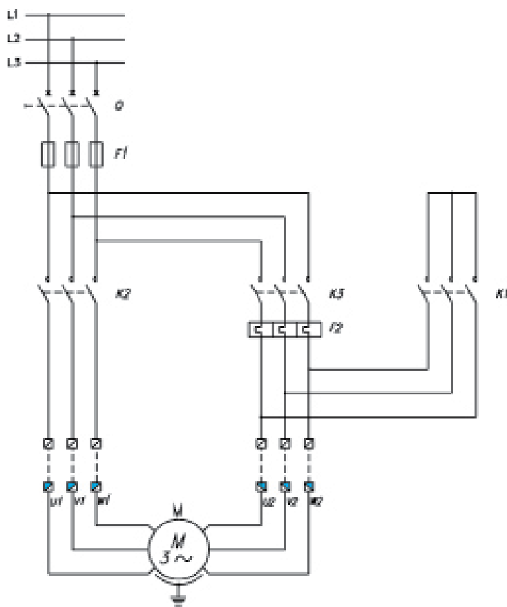
Figura 4. Circuito FM de arranque estrella-triángulo
