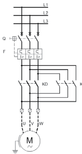
Figura 8. Circuito FM de inversión de marcha
