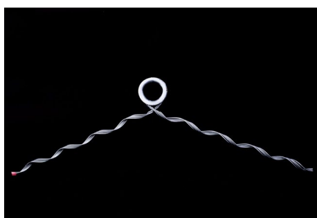
Preformado de suspensión con aro guarda cabo
